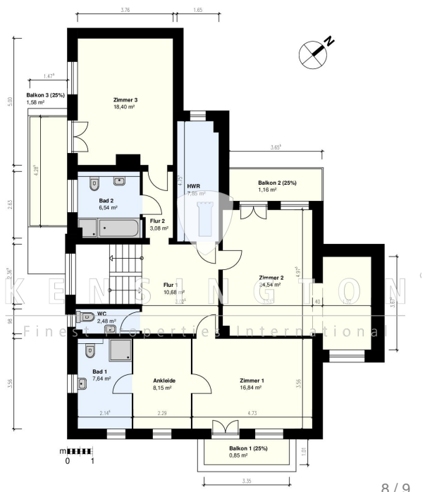
Grundriss OG
